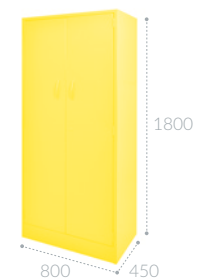
Gabinete universal ligero metálico CODIGO MEMOSA E06B12 CLAVE INIFED MC-M-0027
