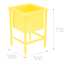
Vertedero con estructura CODIGO MEMOSA E06B32
