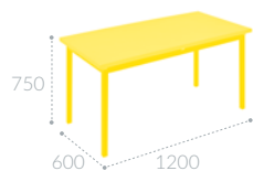
Mesa rectangular con cubierta de polipropileno CODIGO MEMOSA E06B02
