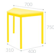
Mesa trapezoidal individual con cubierta de polipropileno de 4to. a 6to. grado CODIGO MEMOSA E06B31
