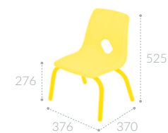
Silla infantil metálica con concha de polipropileno CODIGO MEMOSA E06B06
