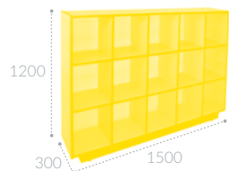
Librero de mdf cubierto de laminado plástico CODIGO MEMOSA E06B15
