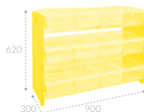
Mueble modular para guarda de material didáctico 12 contenedores CODIGO MEMOSA E06B13
