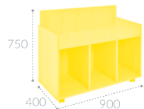
Exhibidor de libros una cara de mdf cubierto de laminado plástico CODIGO MEMOSA E06B14
